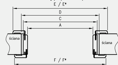
Przekrój poprzeczny TUN
