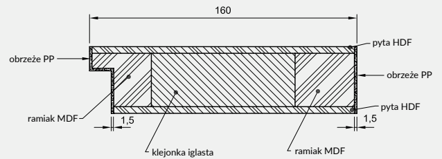
PRZEKRÓJ RAMIAKA PIONOWEGO
