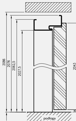
Przekrój poprzeczny alternatywny sposób montażu
