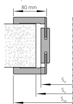
Tunel ZN z opaskami DUO „80”
