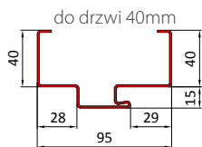
do drzwi 40mm
