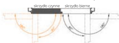
C. Drzwi lewe otwierane na zewnątrz
