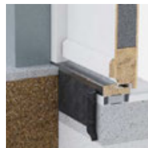
system bazowy (próg)
