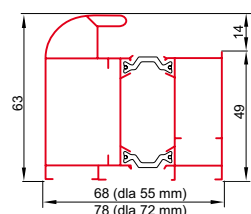
ościeżnica aluminiowa z przegradą termiczną
