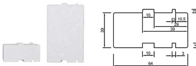
WKŁADKA TERMICZNA POD PRÓG ALUMINIOWY szerokość 100 mm wysokość 30 mm
