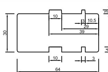
WKŁADKA TERMICZNA POD PRÓG ALUMINIOWY
