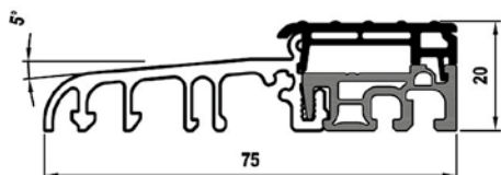
PRÓG ALUMINIOWY Z WKŁADKĄ TERMICZNĄ
