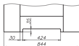
skrzydło SEMPRE „80” z podcięciem wentylacyjnym IMPULS W13
