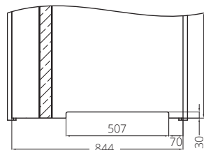
skrzydło IMPULS W13 „80” z podcięciem wentylacyjnym
