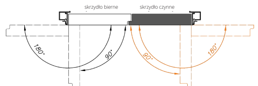
D. Drzwi prawe otwierane na zewnątrz
