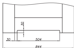
skrzydło ARCO „80” z podcięciem wentylacyjnym
