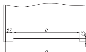
skrzydło FIORD / IMPULS z podcięciem wentylacyjnym
