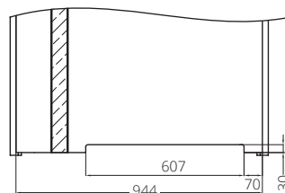
skrzydło IMPULS W13 „90” z podcięciem wentylacyjnym
