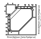
Rysunek techniczny
