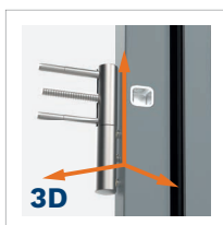
Zawiasy 3D z nasadkami, regulacja w 3 płaszczyznach
