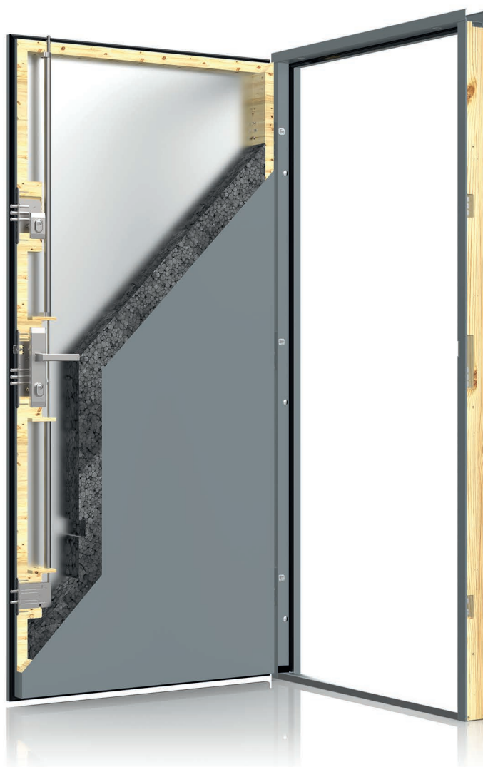
Podwalina podprogowa Ościeżnica Duotherm - opcja Ościeżnica Alutherm - standard
