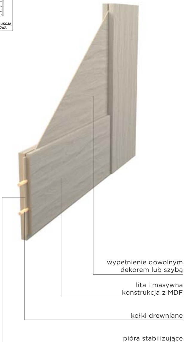
KONSTRUKCJA DREWNIANA
