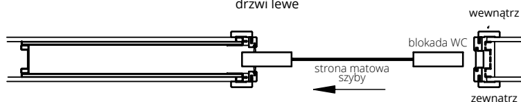
SYSTEM PRZESUWNY DO ZABUDOWY W ŚCIANIE
