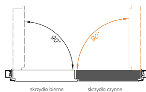
A. Drzwi lewe otwierane do wewnątrz
