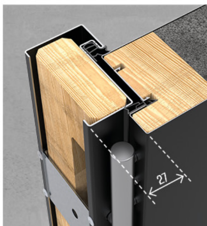
OŚCIEŻNICA DUOTHERM 75
