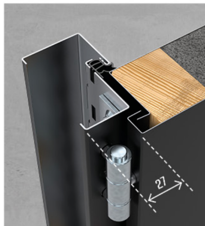
OŚCIEŻNICA PERFOTHERM 60
