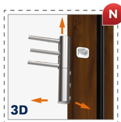
Zawiasy 3D z nasadkami w kolorze okuć*
