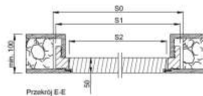
Przekrój E-E drzwi z odwrotną przylgą
