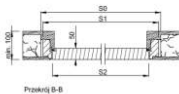
Przekrój B-B drzwi bezprzylgowe
