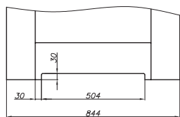
skrzydło ARCO / VERIMO „80” z podcięciem wentylacyjnym
