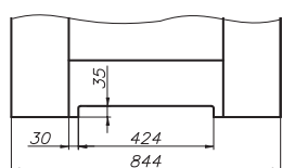
skrzydło SEMPRES „80” z podcięciem wentylacyjnym
