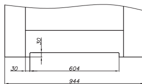
skrzydło ARCO / VERIMO „90” z podcięciem wentylacyjnym
