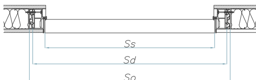
Drzwi Harmony Invest otwierane na zewnątrz pod zabudowę panelową
