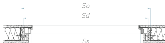
Drzwi Harmony Invest otwierane do wewnątrz pod zabudowę panelową
