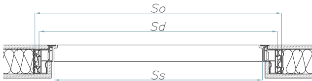
DRZWI OTWIERANE DO WEWNĄTRZ ODZ
