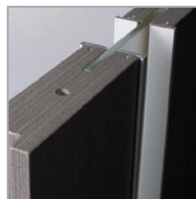
górna przylga w systemie bezprzylgowym
