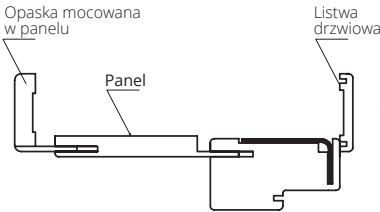
do drzwi B-30, C-30, RC3
