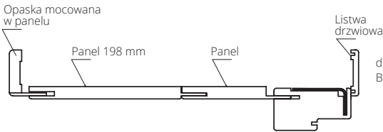
do drzwi CERBER PLUS
