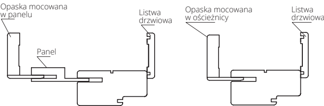
do drzwi CERBER PLUS
