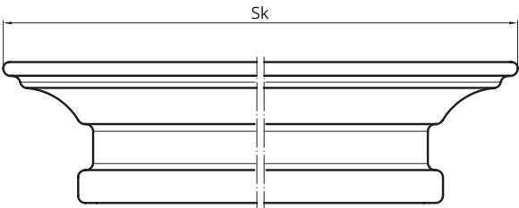
korona do drzwi jednoskrzydłowych przylgowych na jedną stronę
