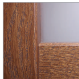
połączenie ramiaka i szyby
